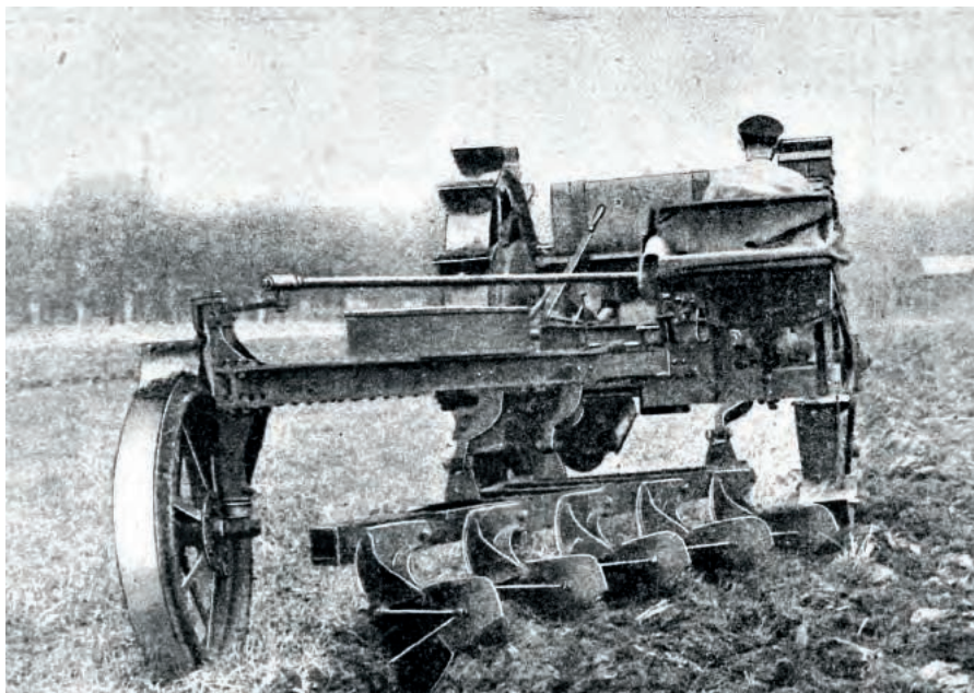
Motorový pluh Wikov, č. neg. 53059-a11710
