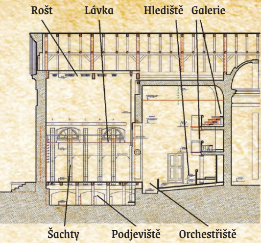
Divadlo z profilu: hlediště je u orchestřiště 11 metrů široké, jeho hloubka je 7 metrů; jeviště má 12 metrů na šířku a 8,5 metrů na hloubku.
